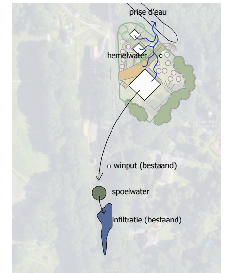
hemelwater naar prise d'eau, verdiepte spoelwatertank bij bestaande infiltratievlen
