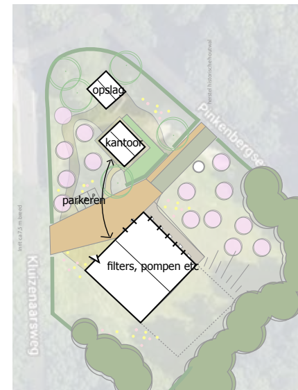
pompen en filter-gebouw, kantoor en opslag
